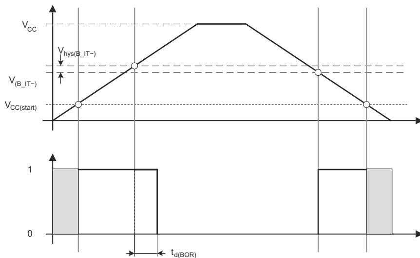
8-9. POR and BOR vs Supply Voltage
