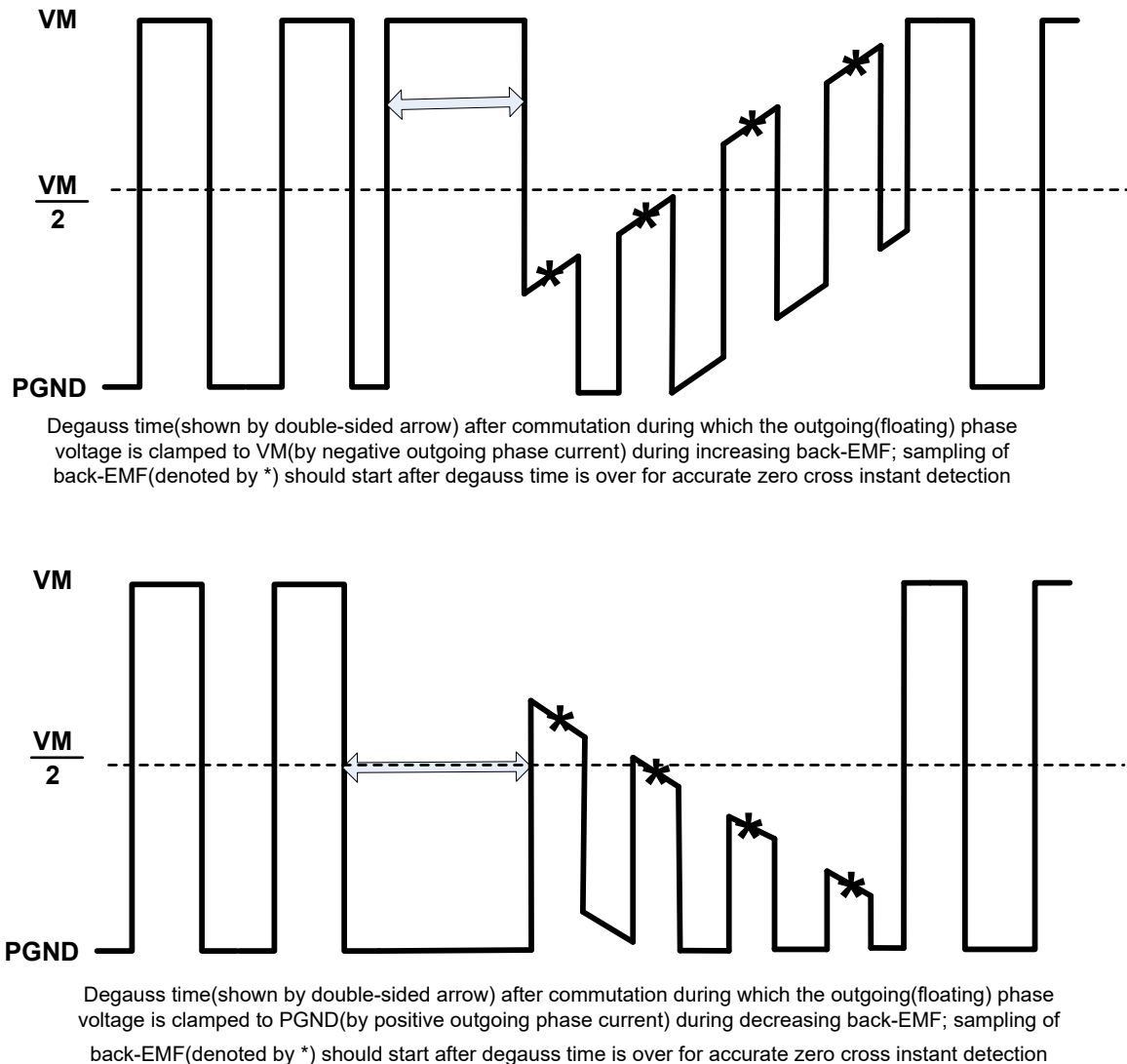
图 8-36. Degauss Time
