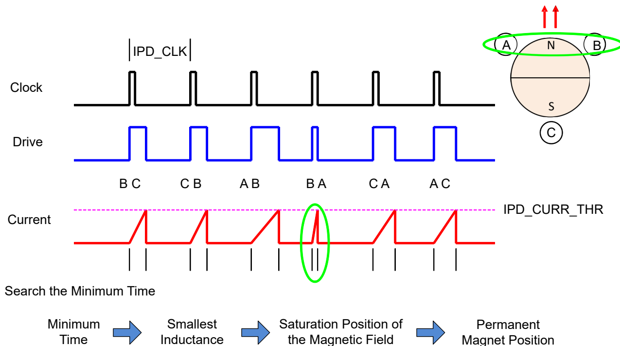
图 7-22. IPD Function
