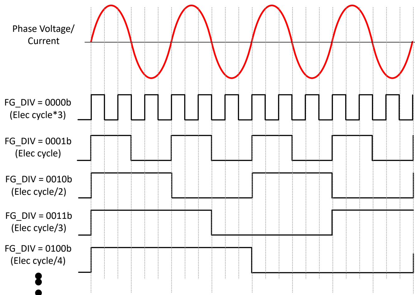
図 6-60. FG 分周器
