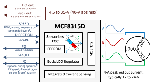
概略回路図
