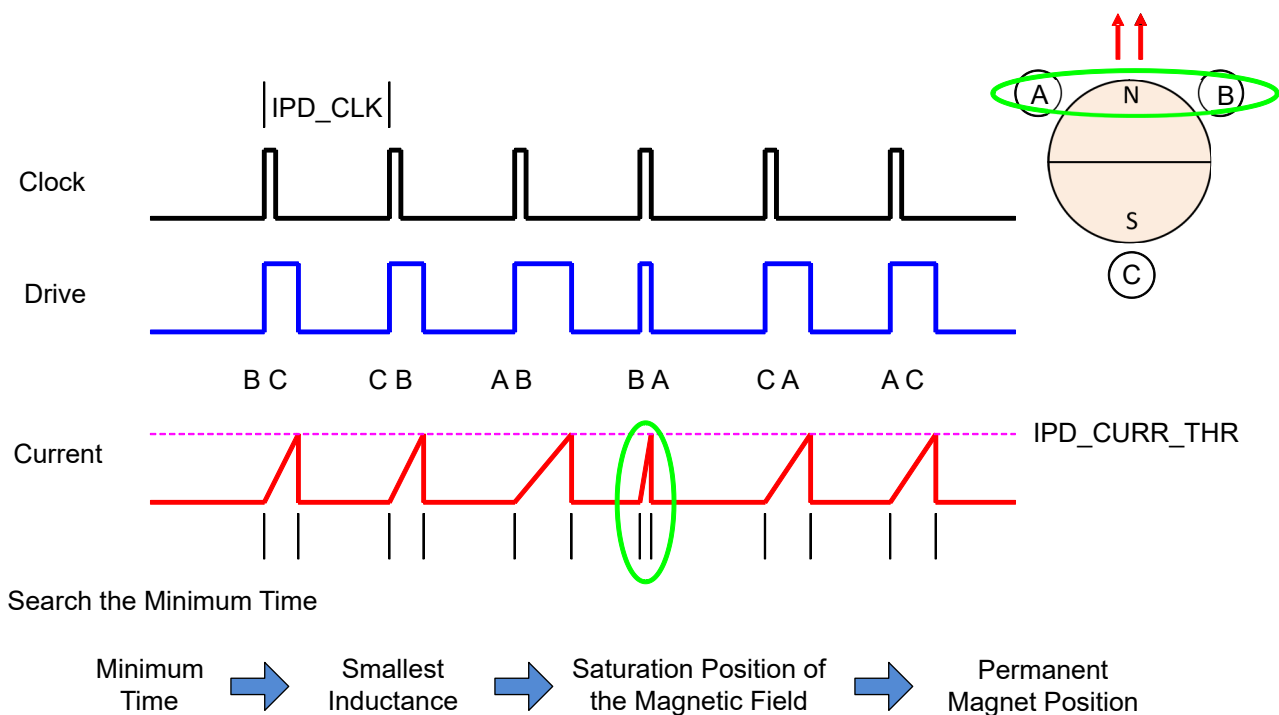
図 6-33. IPD の機能
