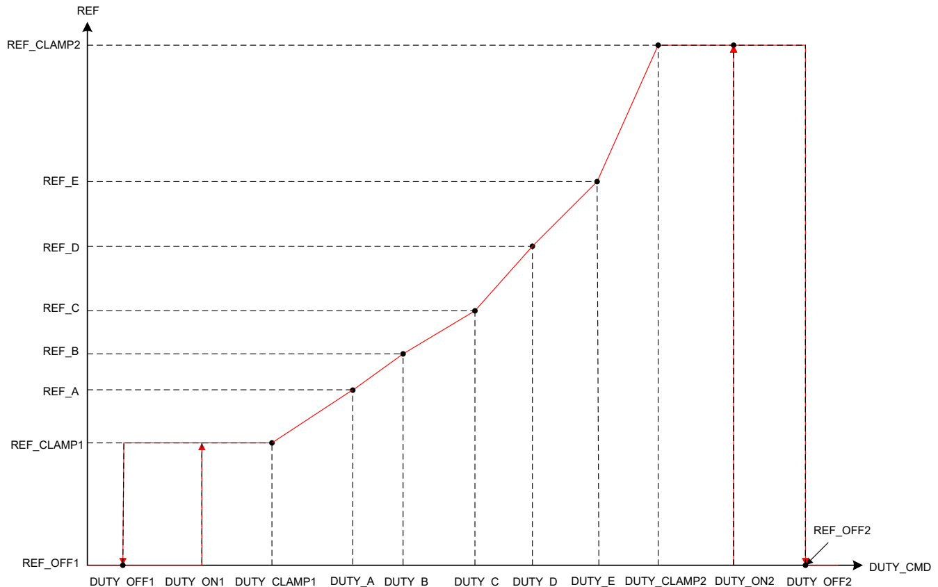
図 6-20. リニア制御プロファイル
