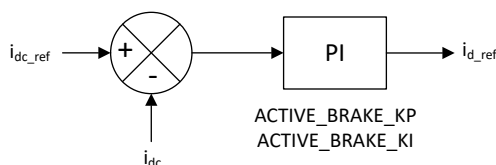
図 6-52. アクティブ ブレーキの i_{d\_ref} 電流制御ループ
