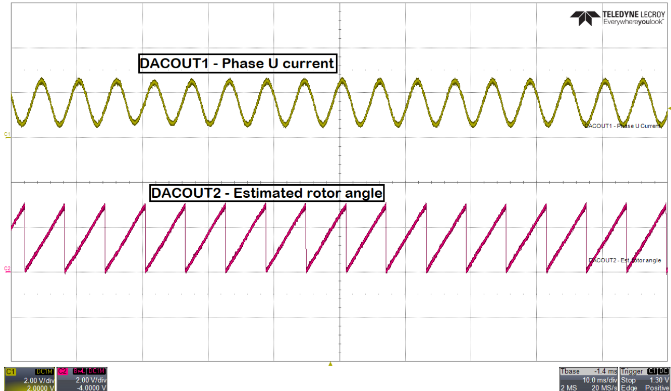
図 9-10. DACOUT1、DACOUT2
