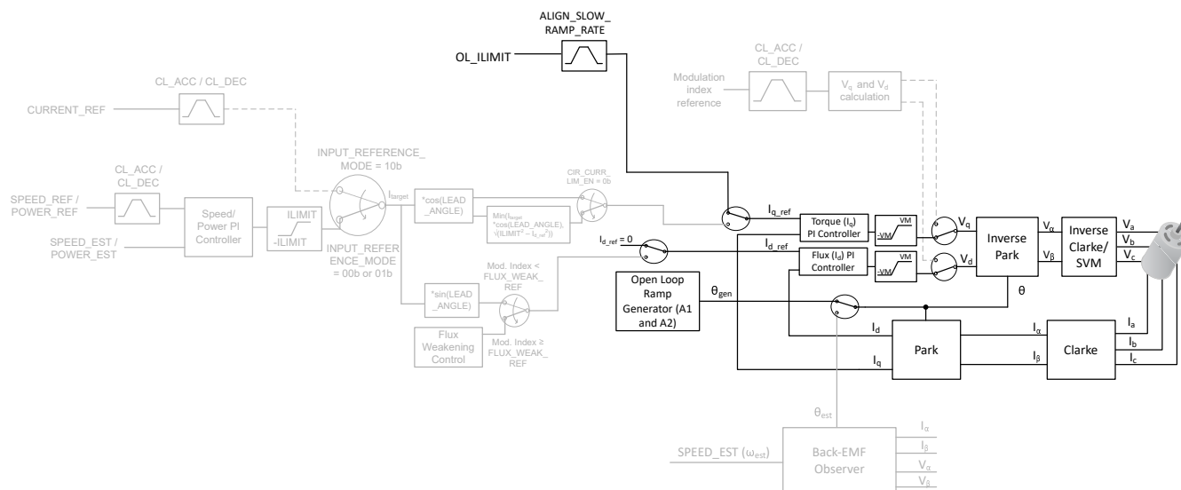
図 6-37. 開ループ
