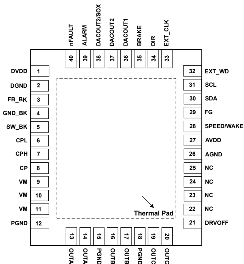
図 4-1. MCF8315D 40 ピン VQFN (露出サーマルパッド付き) 上面図
