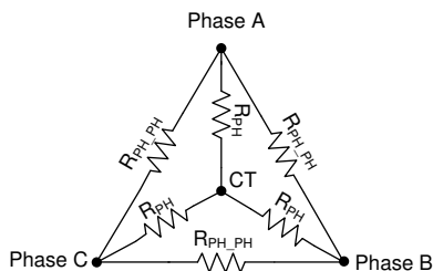
図 6-48. モータ抵抗
