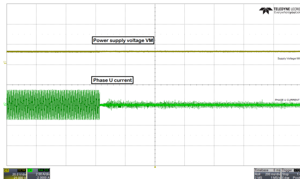
図 9-9. AVS が有効化されている場合の電源電圧と位相電流の波形
