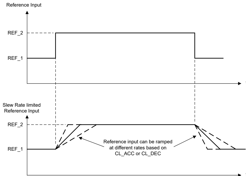
図 6-41. 閉ループ加速 / 減速スルーレート
