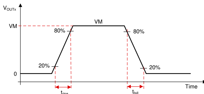
図 6-12. スルーレート タイミング
