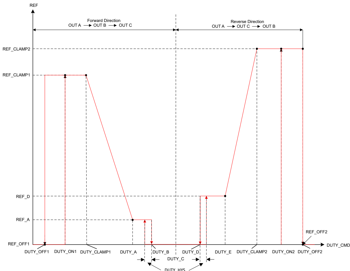
図 6-22. 双方向制御プロファイル
