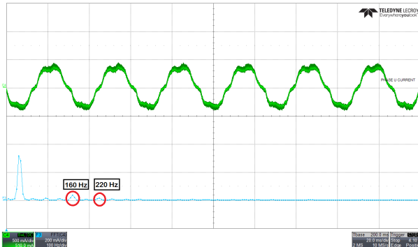
図 9-5. 位相電流と FFT - デッド タイム補償を無効化
