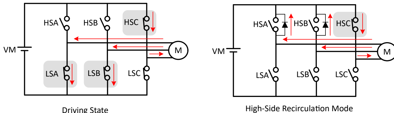
図 6-57. ハイサイド還流
