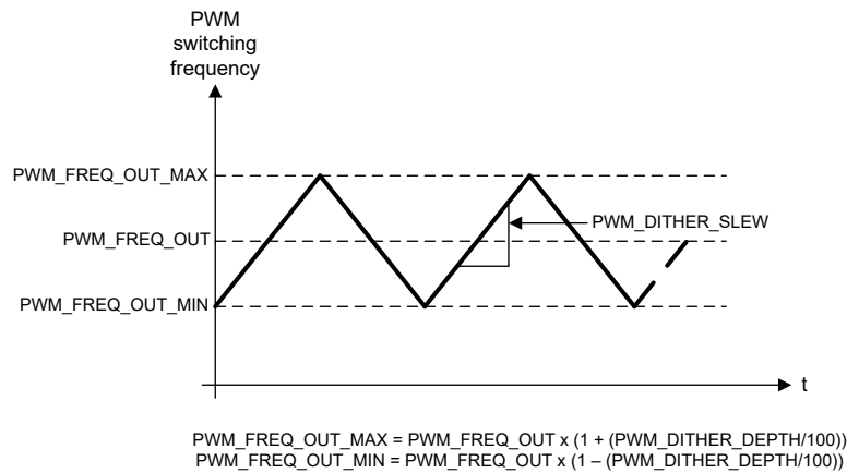
図 6-53. 三角波 PWM ディザリング
