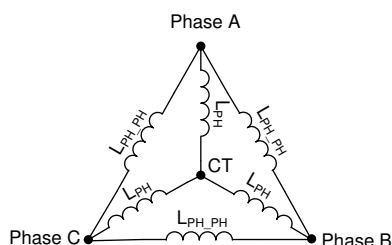
图 7-39. Motor Inductance
