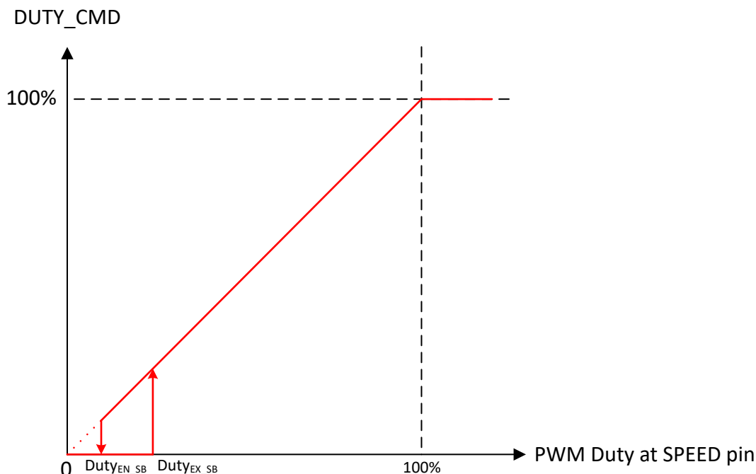
図 7-15. PWM Mode Speed Control
