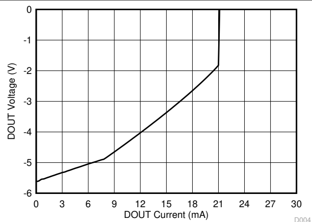
図 5-4. ドライバ VOL と負荷電流との関係
