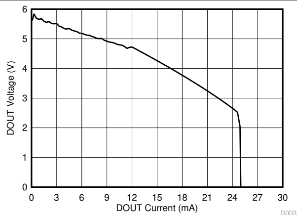
図 5-3. ドライバ VOH と負荷電流との関係
