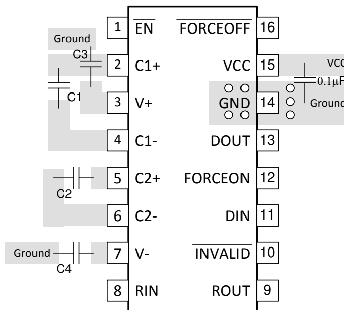
図 8-4. MAX3221E のレイアウト例
