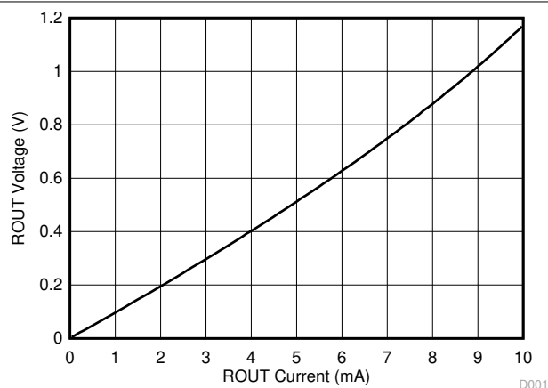
図 5-1. レシーバ VOL と負荷電流との関係
