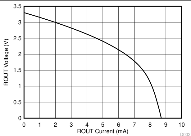
図 5-2. レシーバ VOH と負荷電流との関係
