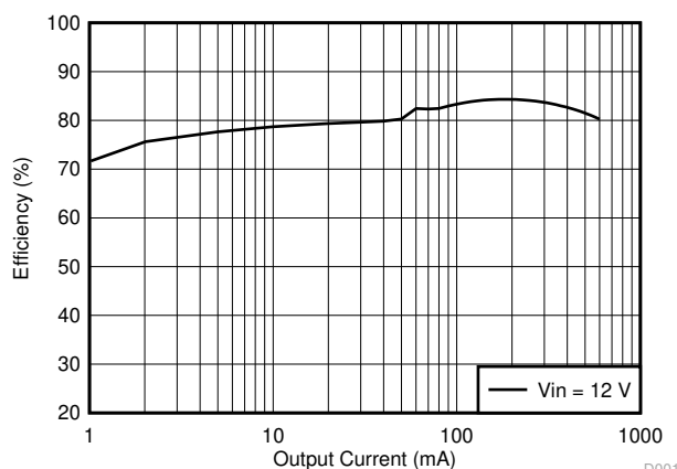
効率と出力電流との関係 ( f_{sw} = 0.7MHz 、 V_{OUT} = 3.3V )
