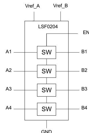
概略回路図
