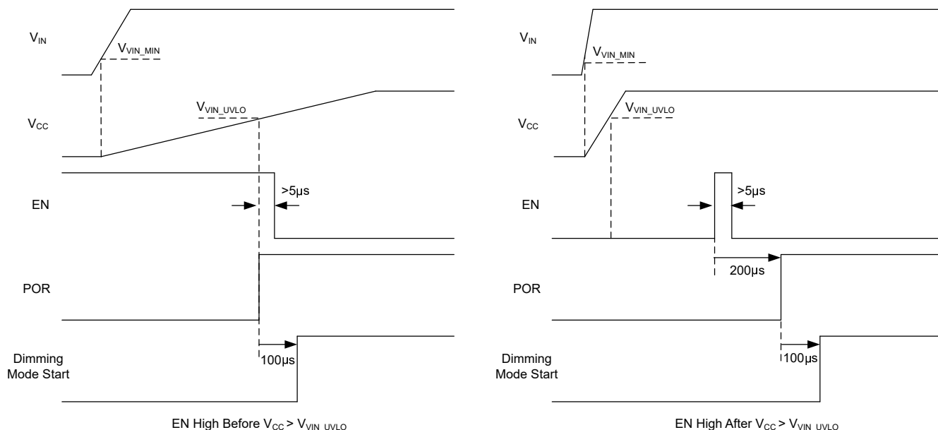
图 7-2. Startup Sequence
