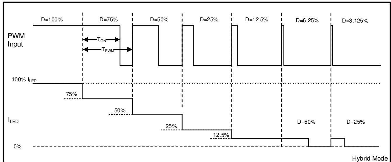
図 7-3. Hybrid Dimming
