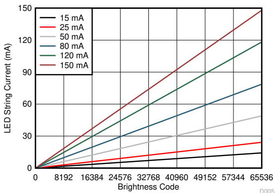
図 5-6. Current Linearity
