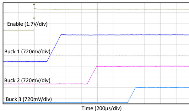
FIG 6-4. Startup, LP876242B0
