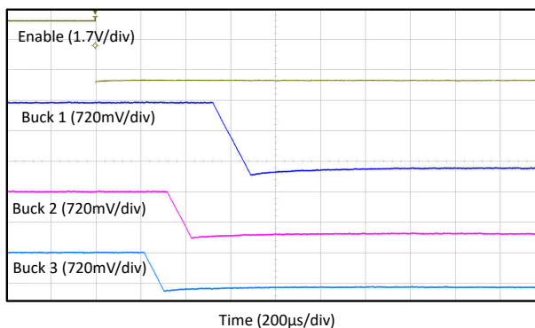
FIG 6-5. Shutdown, LP876242B0
