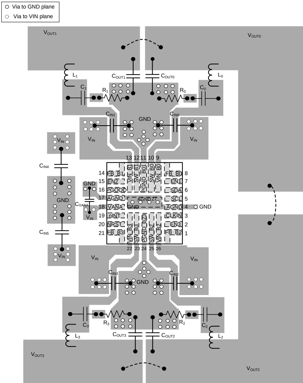
✎ 113. LP8756x-Q1 Board Layout
