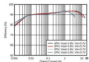
効率と出力電流との関係
