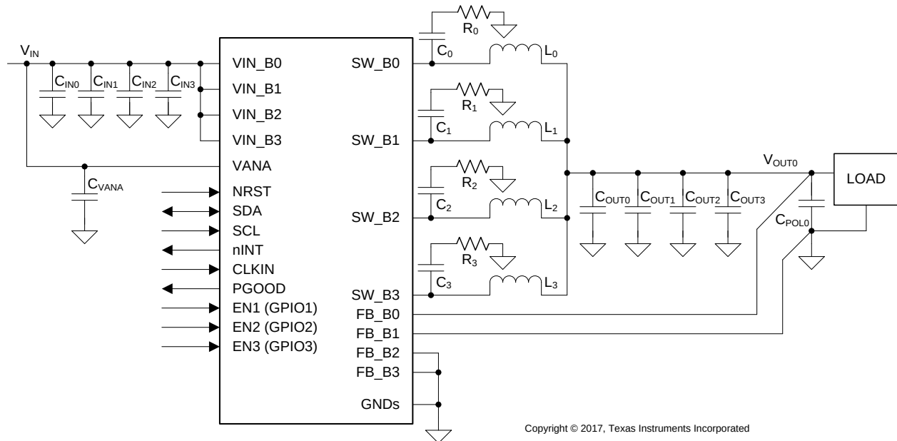
28. 4-Phase Configuration (LP87561-Q1)
