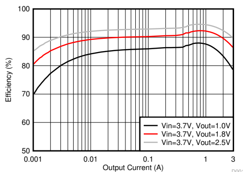
DC/DC 効率と出力電流との関係
