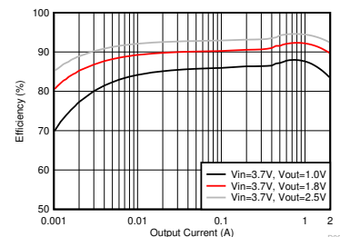
DC/DC 効率と出力電流との関係
