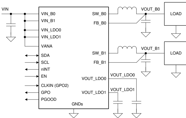
概略回路図
