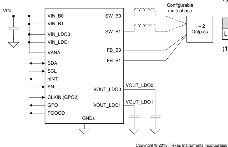
概略回路図
