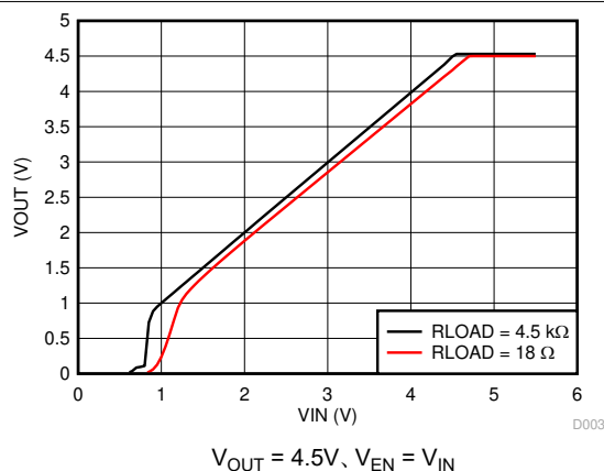
図 5-4. V_{OUT} と V_{IN} の関係
