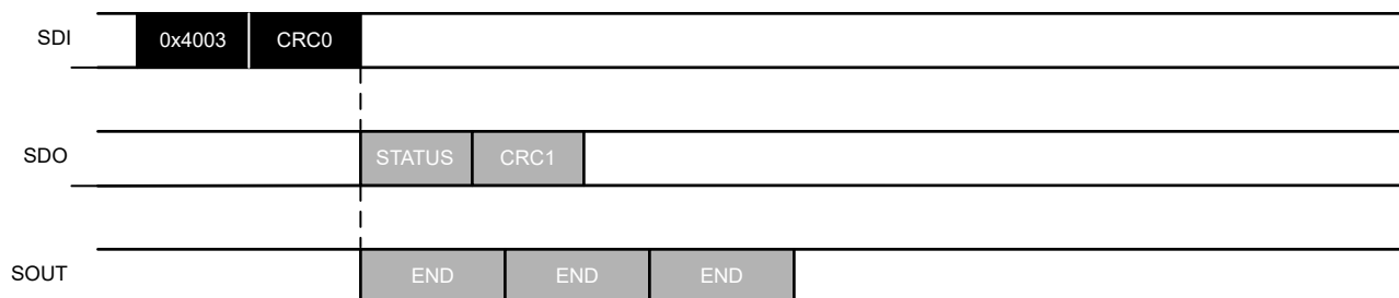
図 7-12. FWD WR END CRC コマンドの例
