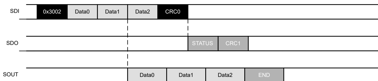
図 7-11. FWD_WR コマンドの例
