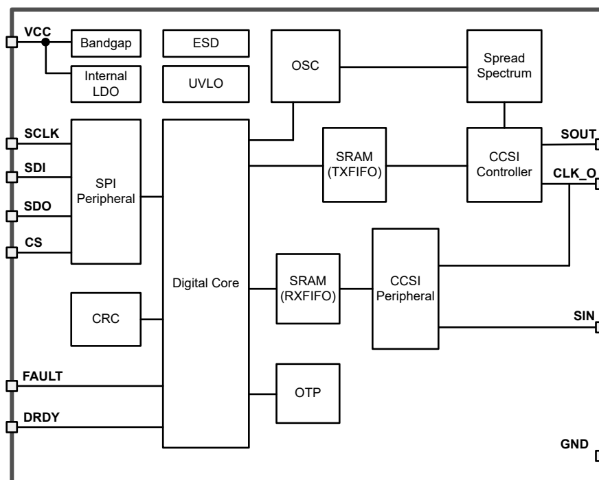
図 7-1. 機能ブロック図
