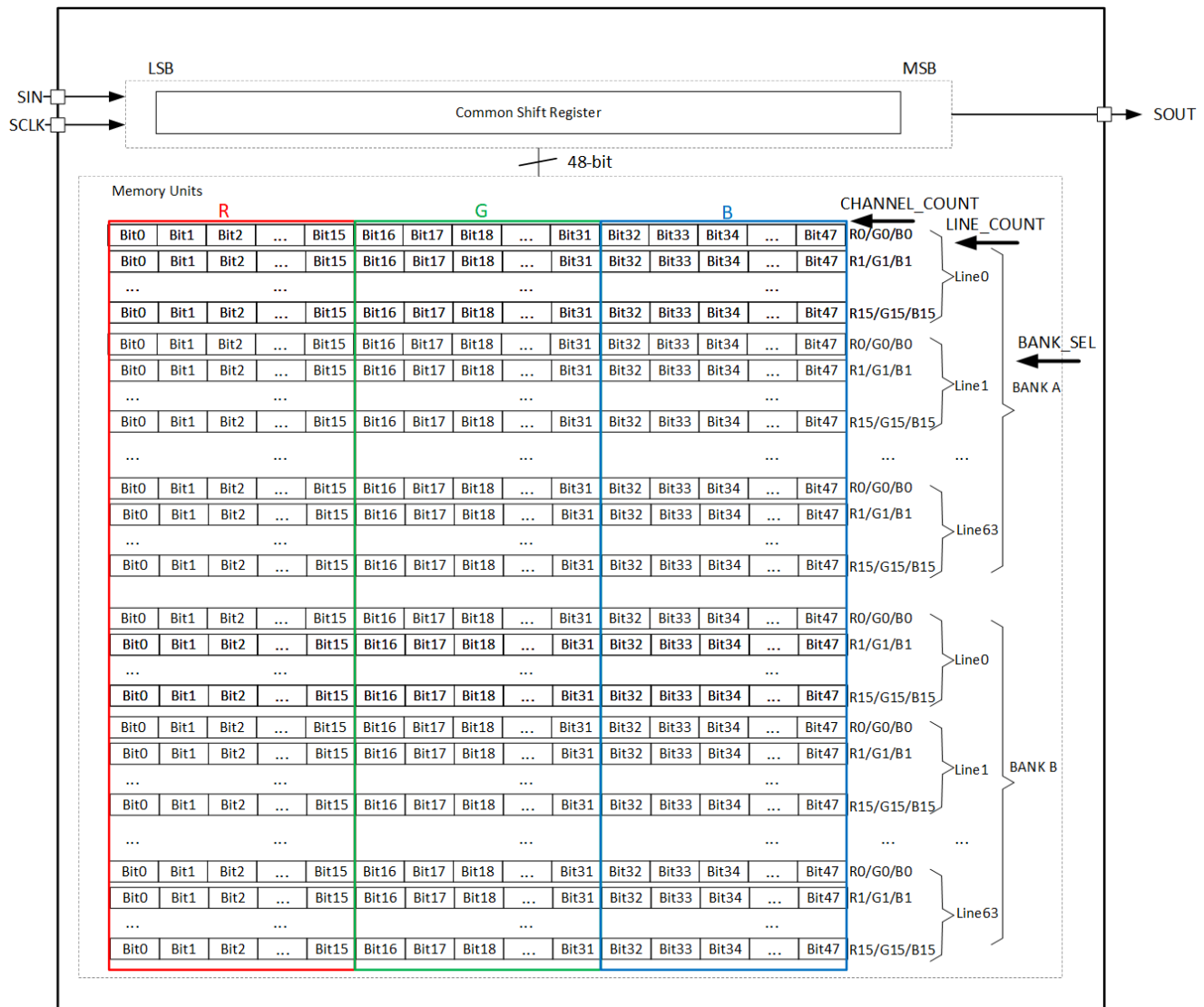
8-27. LP5891-Q1 Memory-unit Structure
