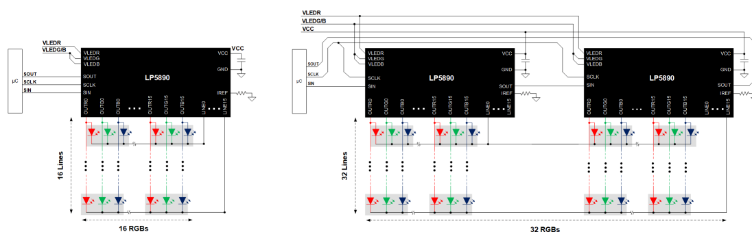
1 デバイスまたは 2 デバイス・スタック接続の LP5890
