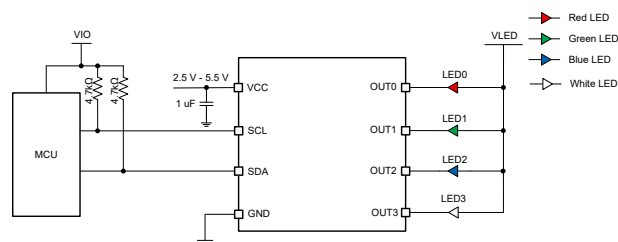
LP5816 の概略回路図
