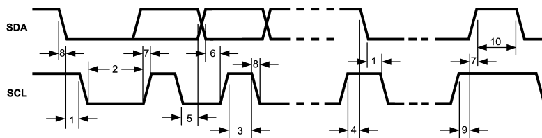
1. Timing Parameters
