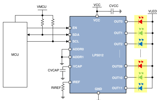
簡略回路図
