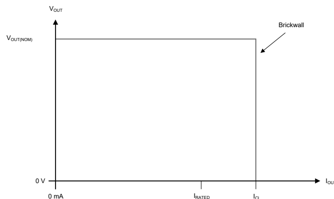
図 6-2. Current Limit
