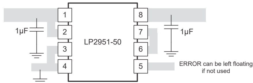
図 7-7. LP2951 Layout Example (D or P Package)
