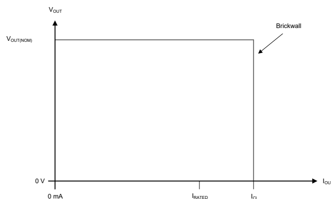
図 6-2. Current Limit
