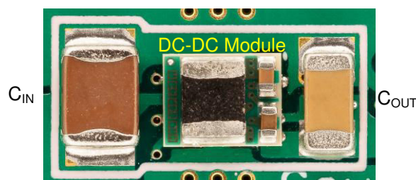
片面レイアウト、ソリューション・サイズの 24V～5V の 0.5A の DC/DC コンバータ
