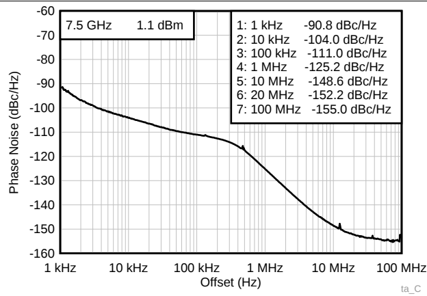
図 93. Direct VCO Noise
