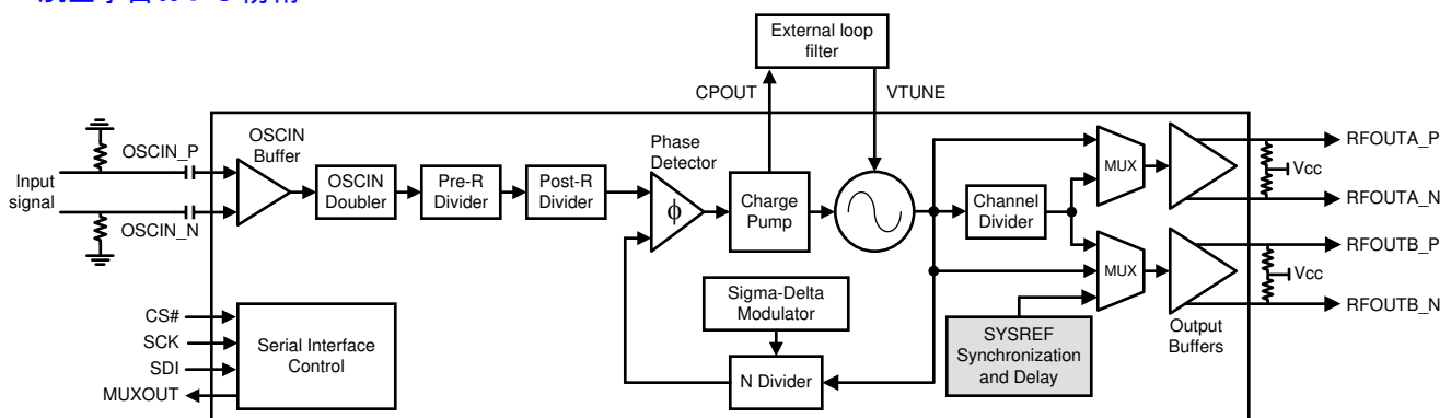
概略回路図
