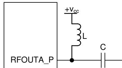
图 8-3. Inductor Pullup
