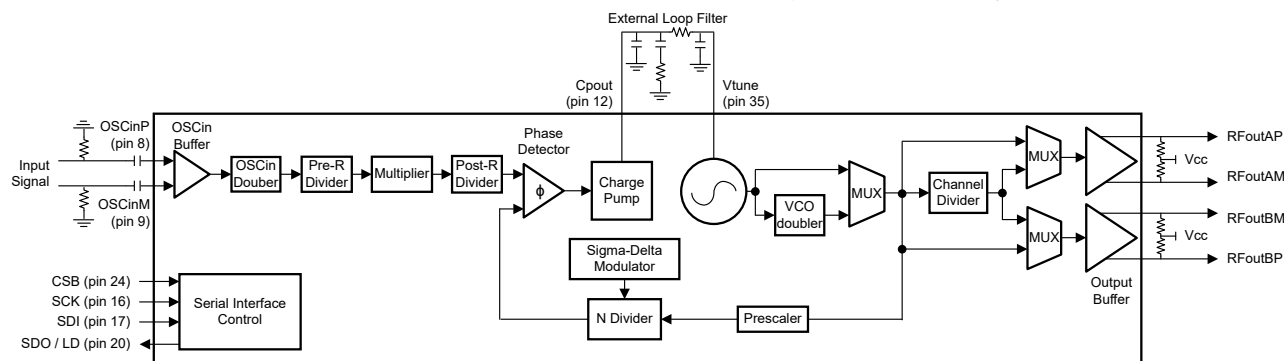
概略回路図
