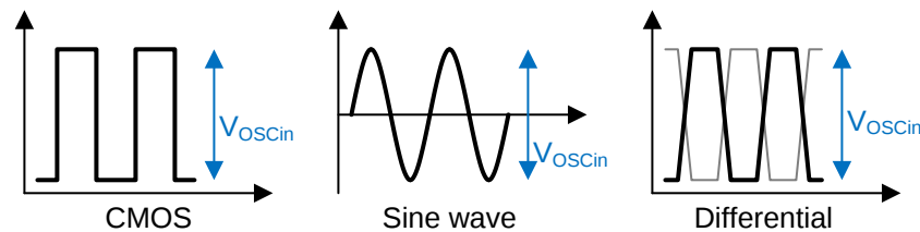
図 154. Input Clock Definition
