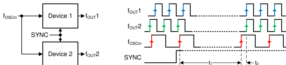
图 33. Phase Synchronization
