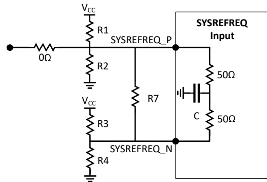
図 8-5. DC 結合、シングルエンド入力
