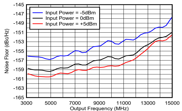
図 5-5. バッファ モードのノイズフロア
