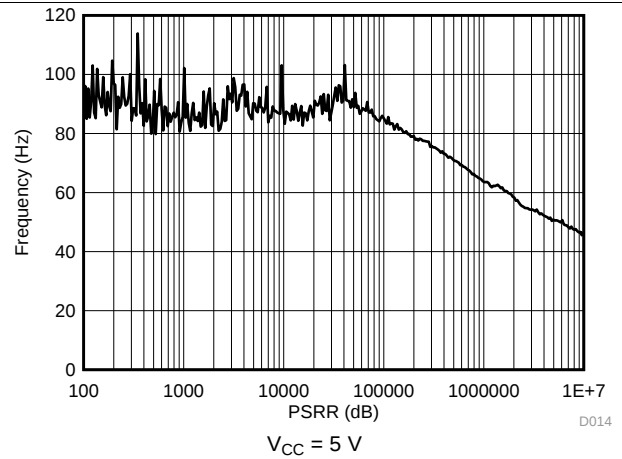
图 14. Psrr vs Frequency
