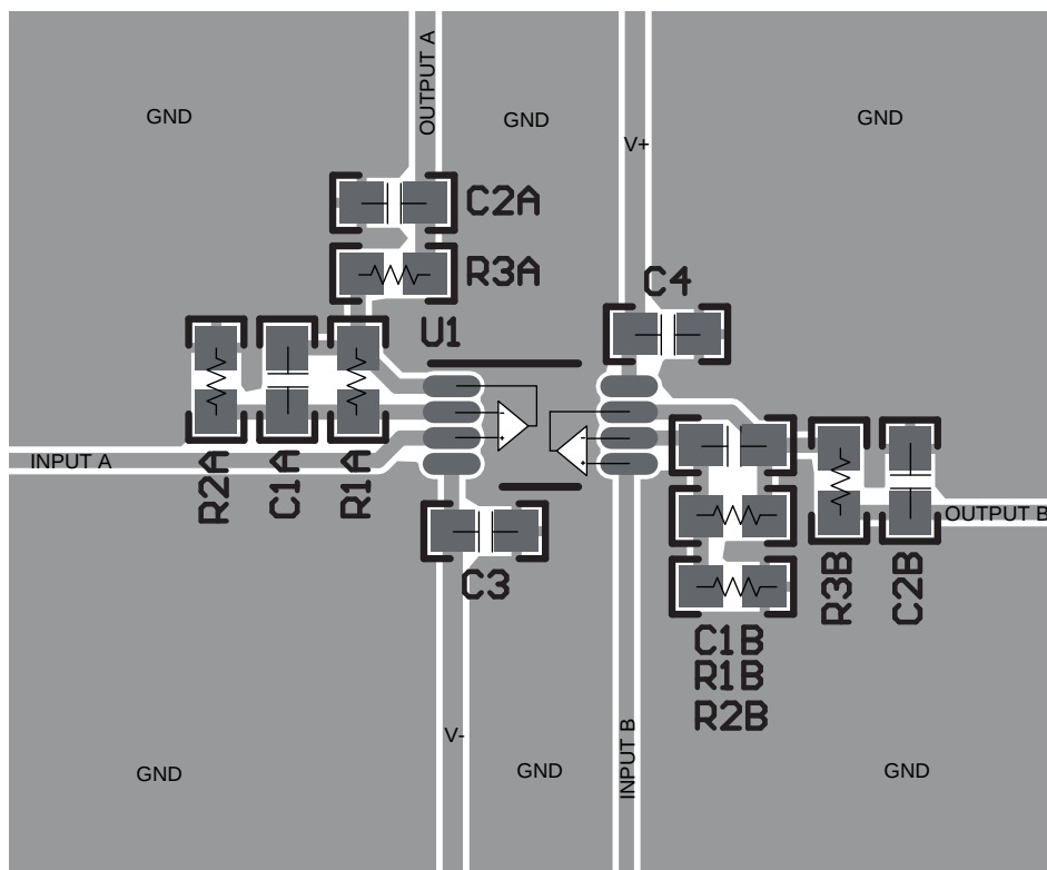
FIG 30. Layout Example
