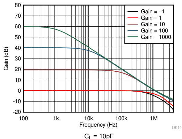
図 5-6. 開ループ・ゲインと周波数との関係
