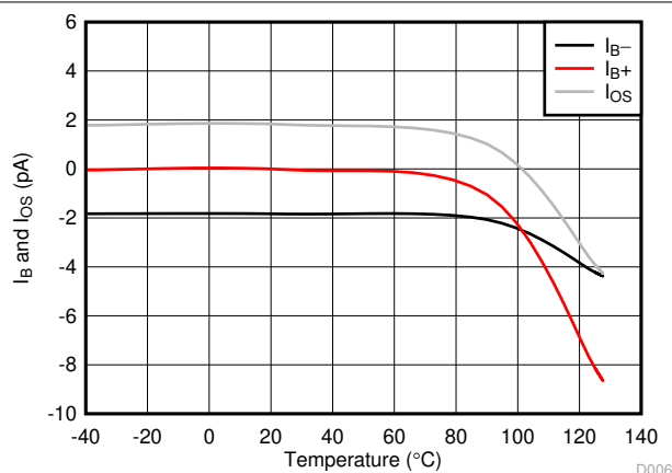
図 5-1. I_B および I_{OS} と温度との関係
