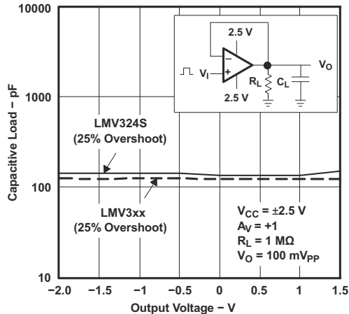
図 6-7. 安定性と容量性負荷との関係
