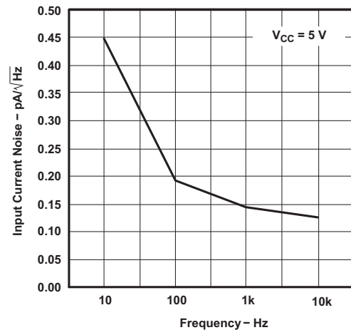
図 6-40. 入力電流ノイズと周波数との関係
