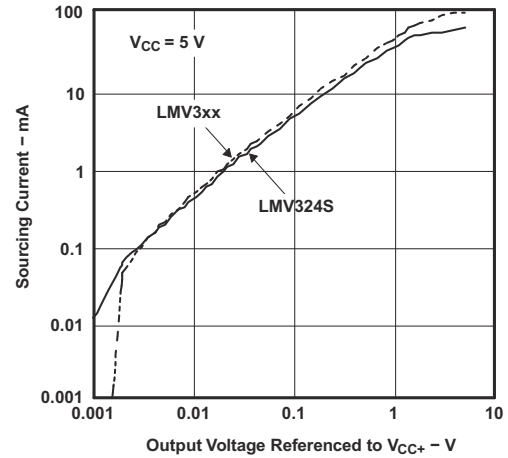
図 6-14. ソース電流と出力電圧との関係
