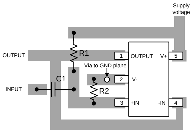
Figure 25. LMV116/LMV118 Layout
