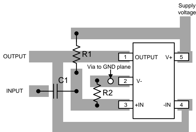
Figure 25. LMV116/LMV118 Layout
