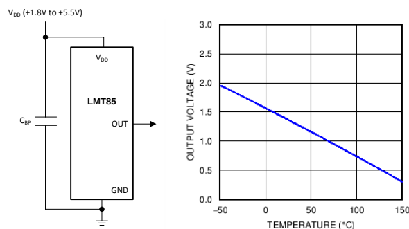
出力電圧と温度との関係
