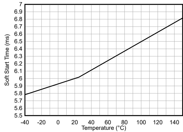
図 6-6. Soft-Start Time
