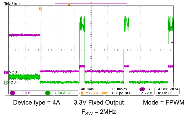
図 8-9. Short-Circuit Applied
