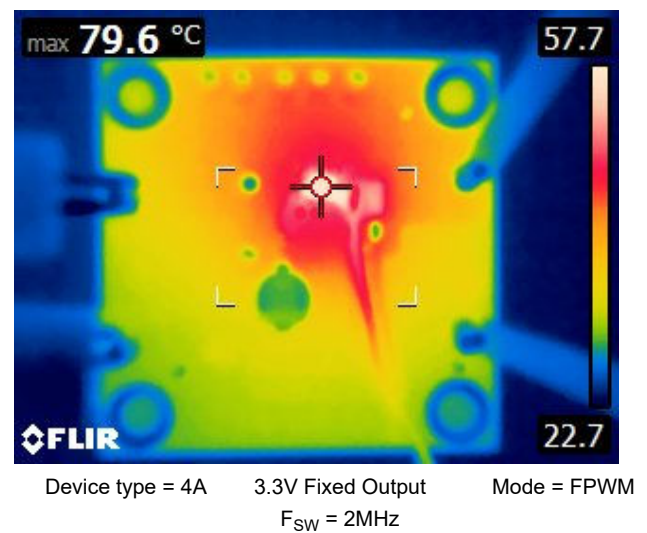
図 8-11. Thermal Performance
