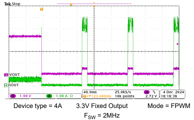
図 8-9. Short-Circuit Applied
