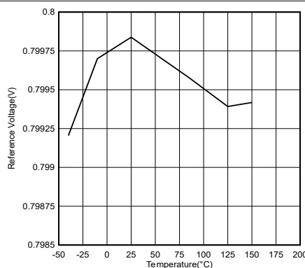
図 6-12. リファレンス電圧と温度との関係
