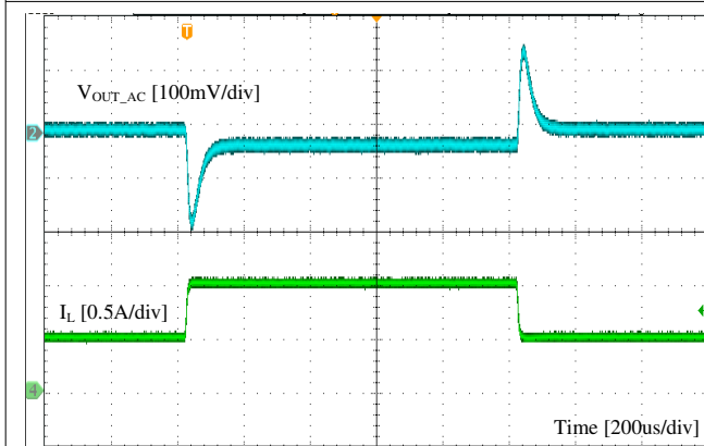
図 8-7. 負荷過渡
