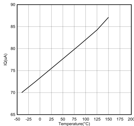
図 6-10. I_Q と温度との関係
