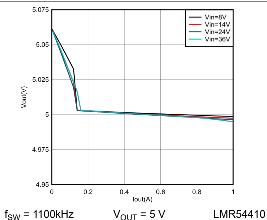
図 6-7. 5-V Load Regulation
