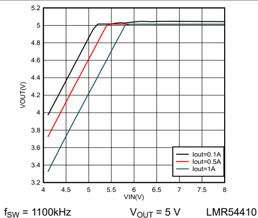
図 6-9. 5-V Dropout
