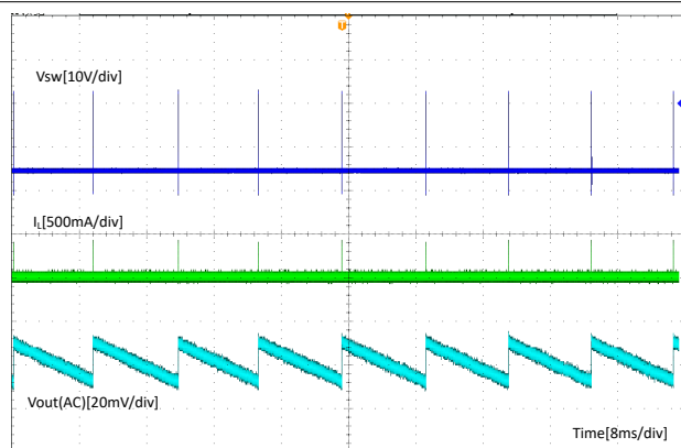
図 8-3. Ripple at No Load
