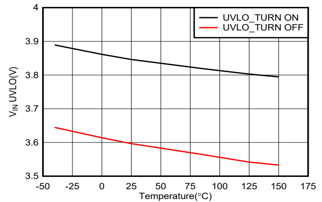
図 6-16. V_{IN} UVLO Versus Temperature
