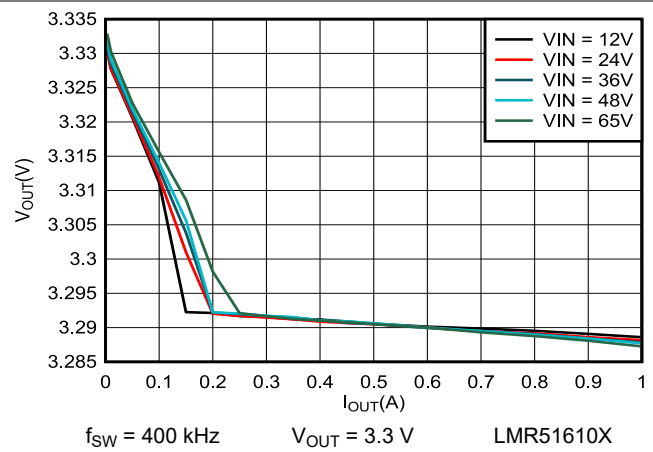
図 6-14. 3.3-V Load Regulation
