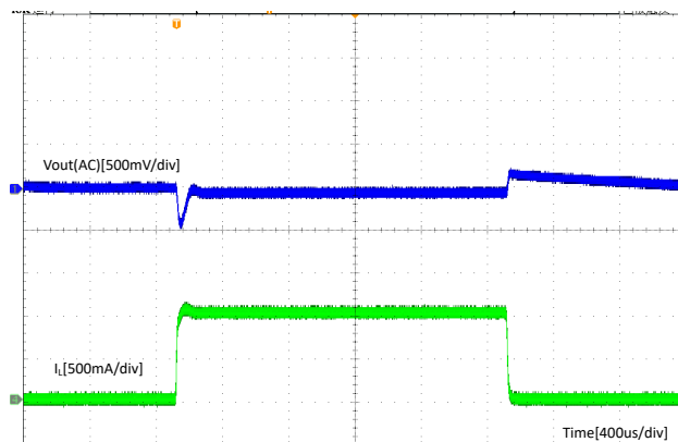
図 8-8. Load Transient (0 A – 1 A)
