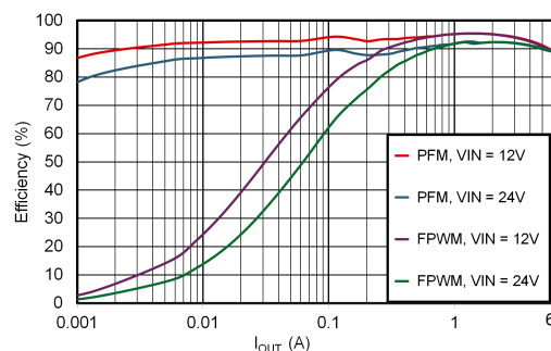
効率と出力電流との関係 V_{\text{OUT}} = 5\text{V} 、400kHz
