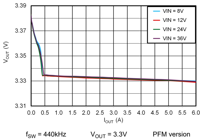
図 6-3. 3.3V Load Regulation
