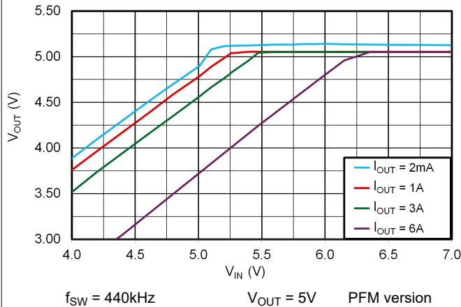
図 6-5. 5V Dropout
