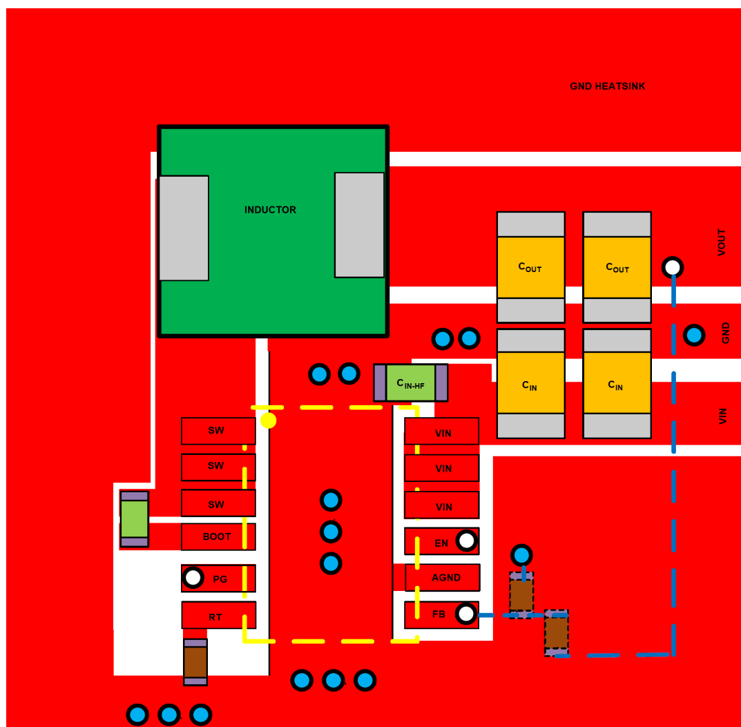
図 8-10. Layout
