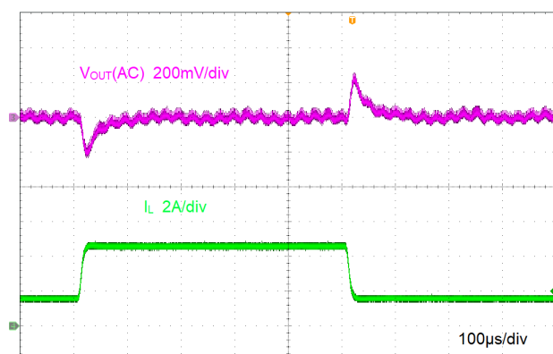
図 8-6. Load Transient
