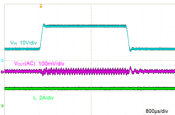
図 8-7. Line Transient
