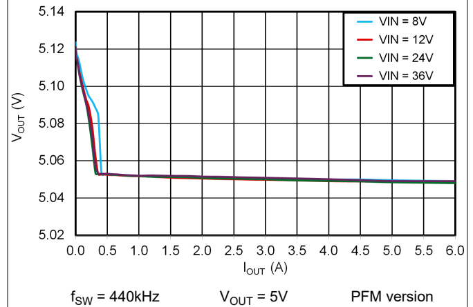
図 6-4. 5V Load Regulation
