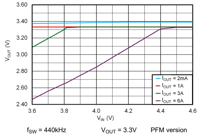
図 6-6. 3.3V Dropout
