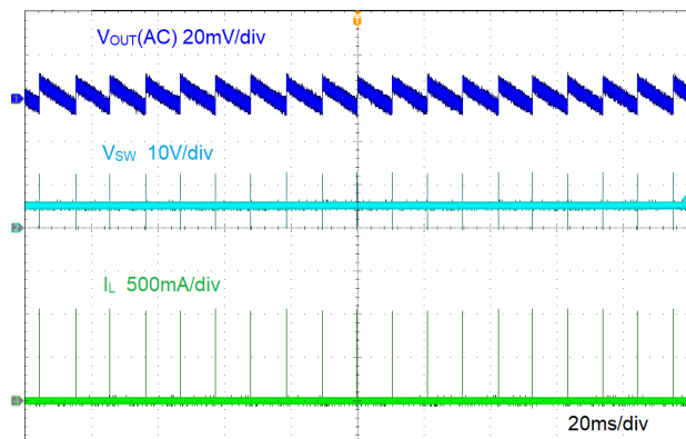
図 8-2. Ripple at No Load
