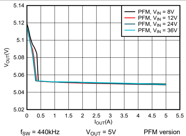
図 6-6. 5V Load Regulation
