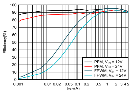
効率と出力電流との関係 V_{\text{OUT}} = 5\text{V} 、 400\text{kHz}
