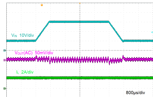
図 8-7. Line Transient
