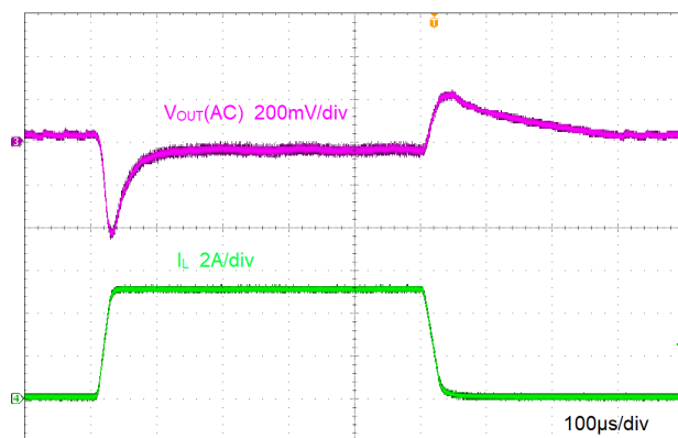
図 8-6. Load Transient
