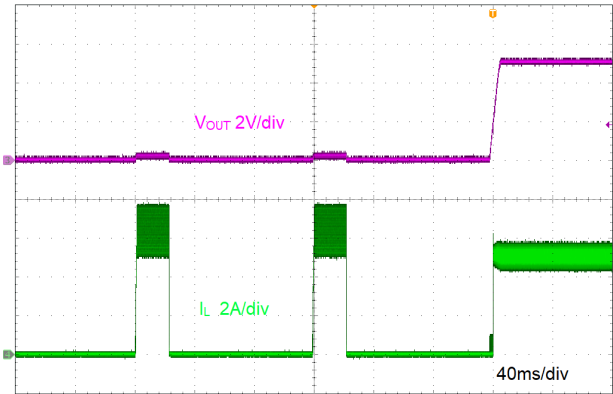
図 8-9. Short Recovery
