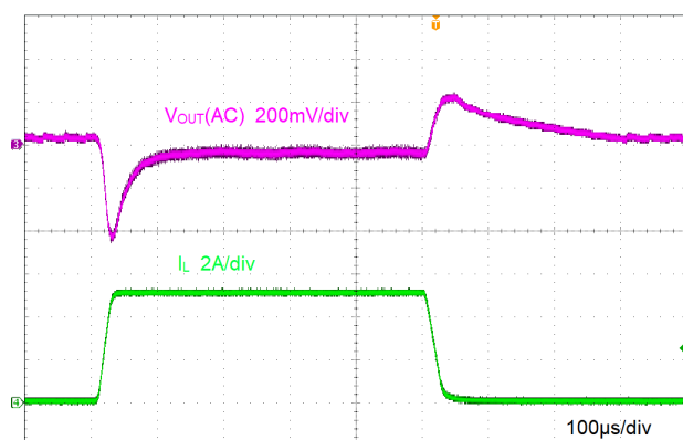
图 9-6. Load Transient
