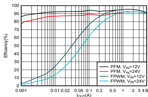
効率と出力電流との関係 V_{OUT} = 5V 、500kHz
