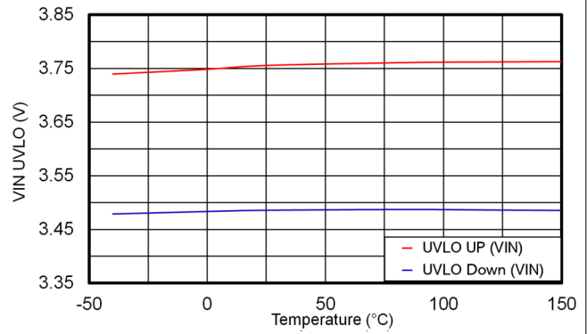
7-10. V_{IN} UVLO
