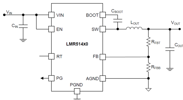
概略回路図
