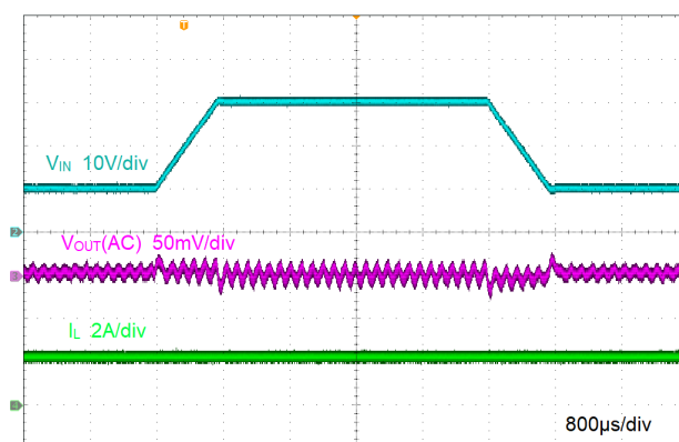
图 9-7. Line Transient
