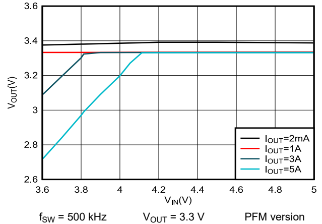
7-8. 3.3-V Dropout
