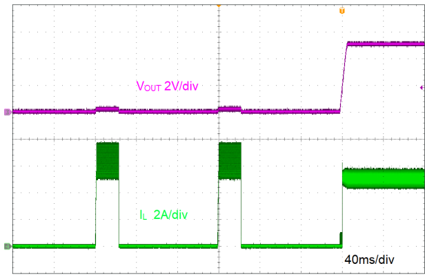
图 9-9. Short Recovery
