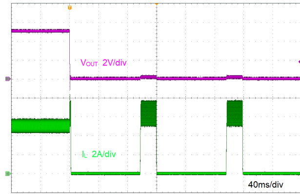
图 9-8. Short Protection
