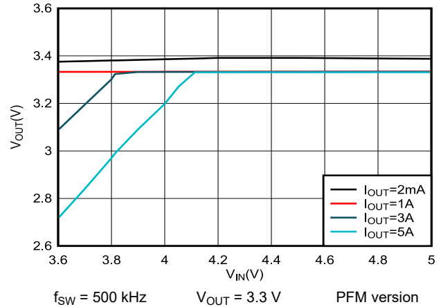
7-8. 3.3-V Dropout
