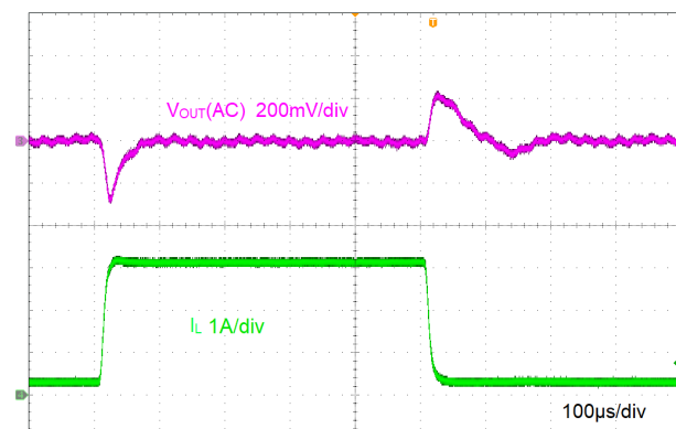
図 8-6. Load Transient
