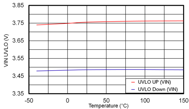
図 6-14. V_{IN} UVLO
