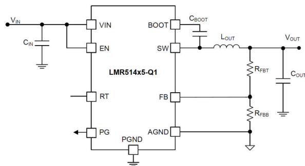
概略回路図
