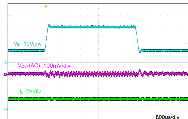
図 8-7. Line Transient
