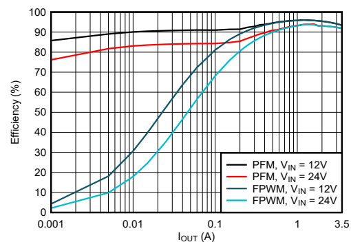
効率と出力電流との関係 V_{\text{OUT}} = 5\text{V} 、440kHz
