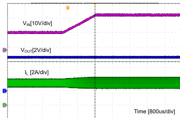
图 9-7. Line Transient
