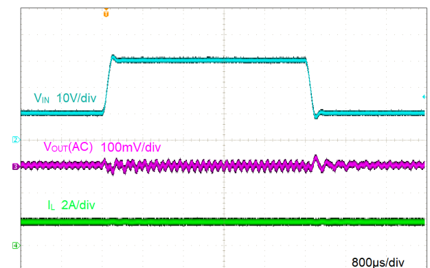
図 8-7. Line Transient
