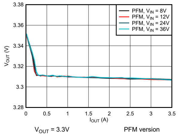
図 6-10. 3.3V Load Regulation
