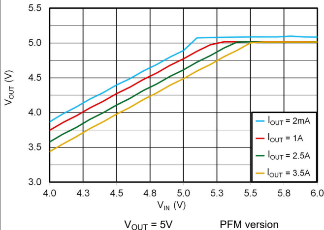
図 6-11. 5V Dropout
