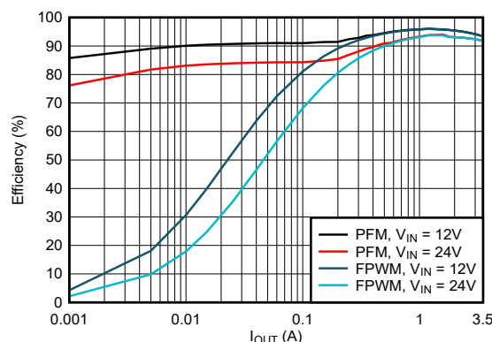
効率と出力電流との関係 V_{OUT} = 5V 、500kHz
