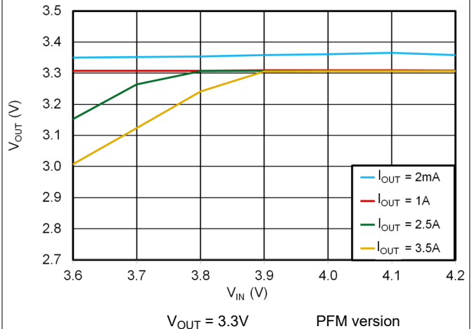
図 6-12. 3.3V Dropout
