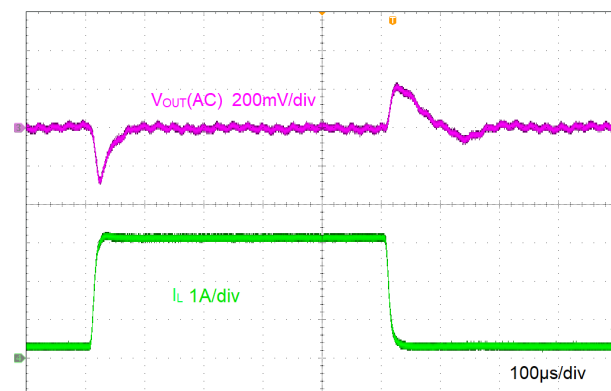
図 8-6. Load Transient
