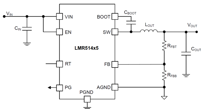
概略回路図
