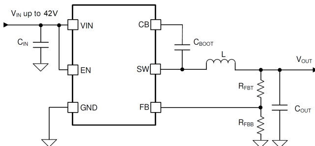
概略回路図
