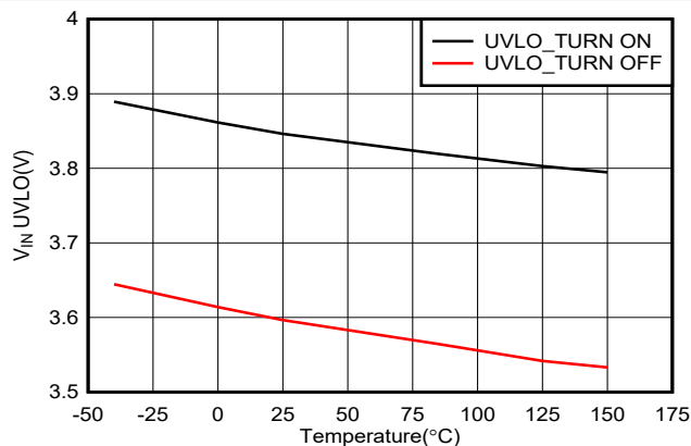
図 6-10. V_{IN} UVLO Versus Temperature
