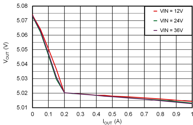
図 6-7. 5V load Regulation
