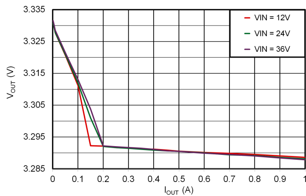
図 6-8. 3.3V Load Regulation
