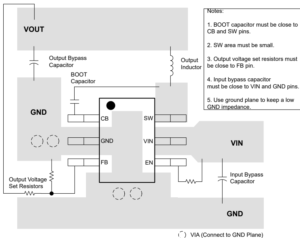
図 8-10. Layout
